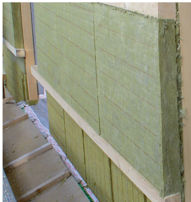
Fig. 6: Fixation par coincement
